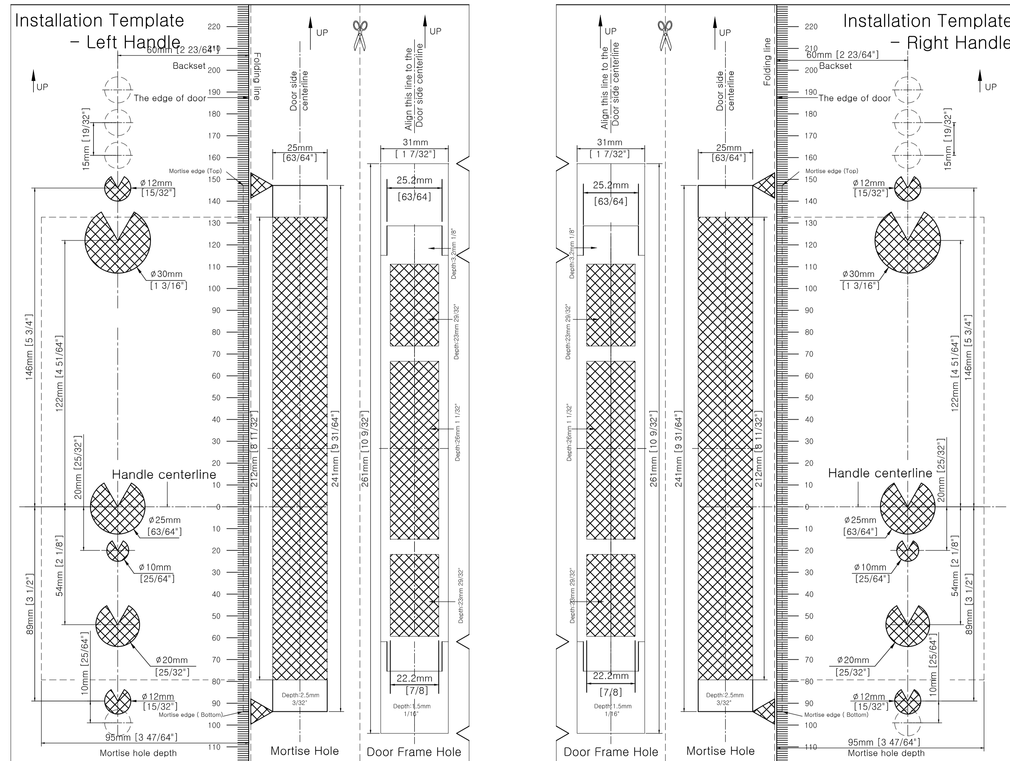
TL100_国标锁体 英文开孔模板
